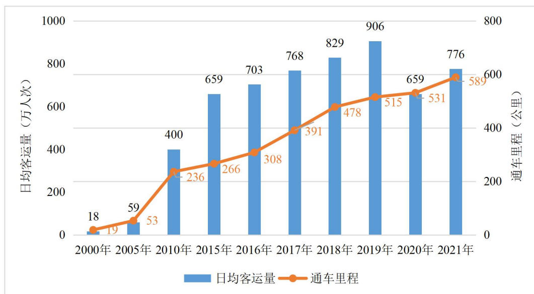
图 5.2 广州地铁线网和客流发展历程
